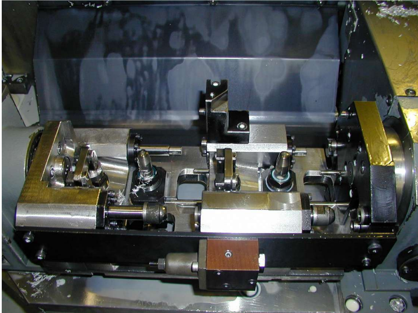
UTILLAJE DOBLE DE AMARRE PARA CENTRO DE MECANIZADO
